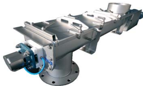
Trogtransporteur met scharnierende deksels welke 100% stofdicht zijn inwendig heerst een overdruk van 200 mbar
